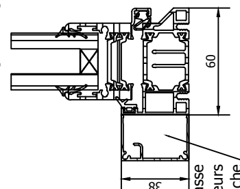
C-C ( 1/2 )
