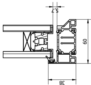
C-C ( 1/2 )
