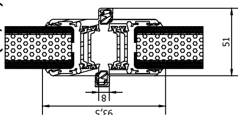
B-B ( 1/2 )
