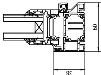
C-C ( 1/2 )
